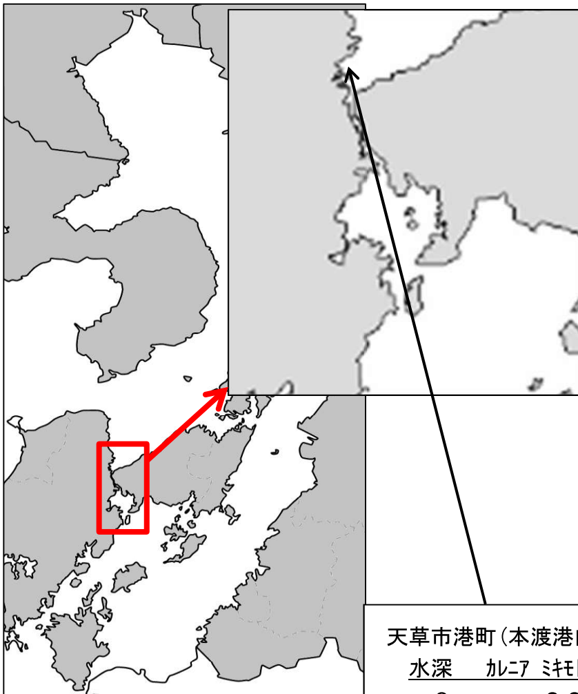
図 調査海域
